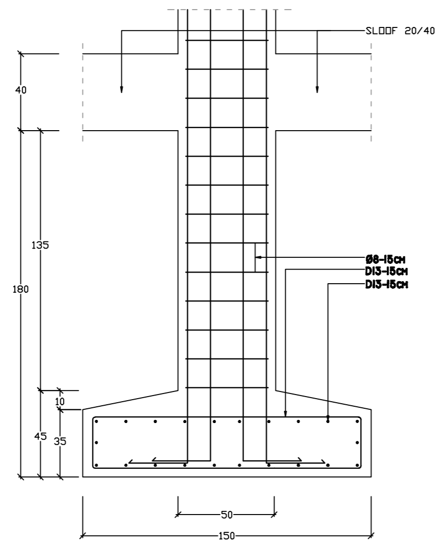
POTONGAN A SKALA 1 : 20
