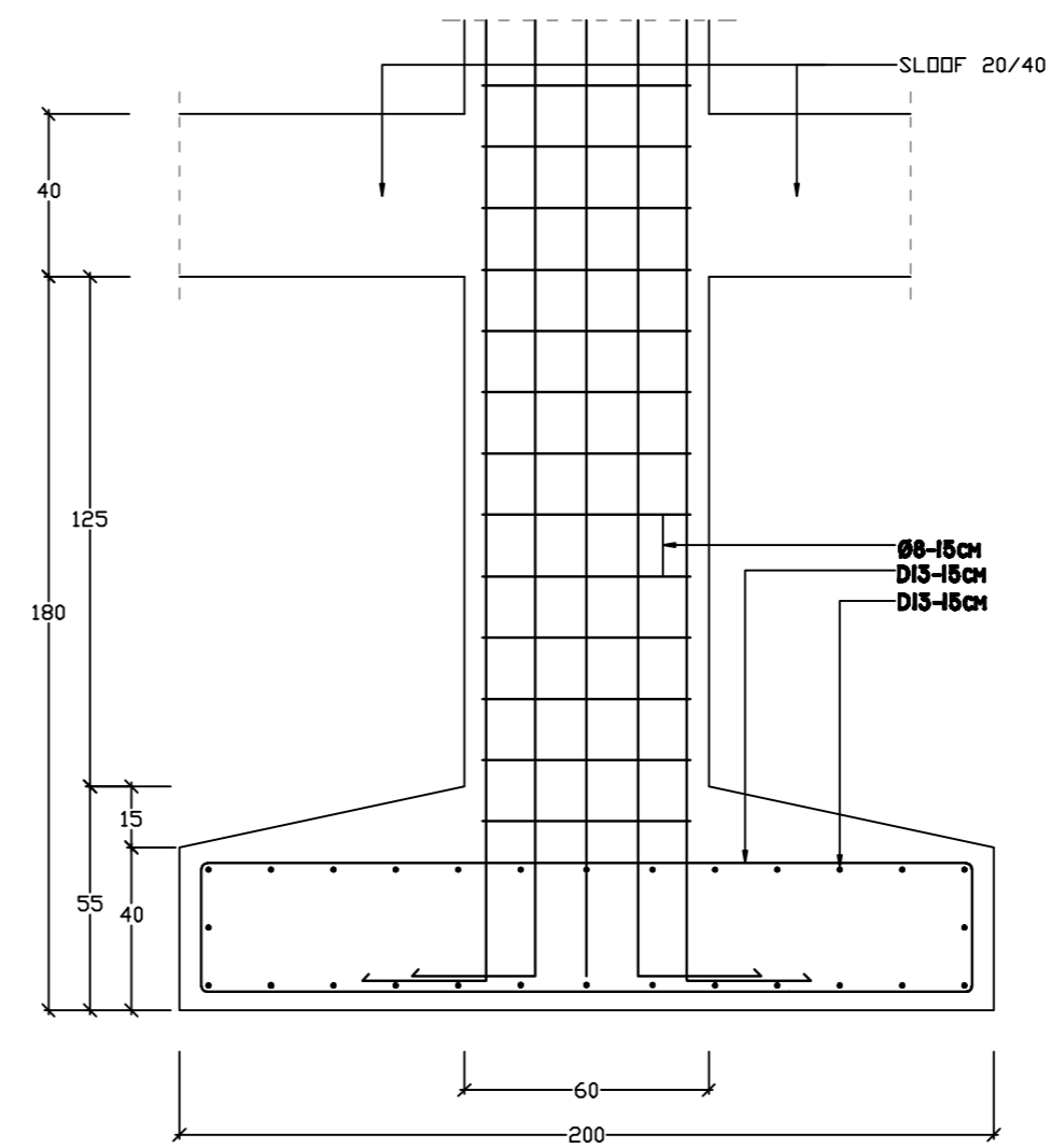
POTONGAN A SKALA 1 : 20
