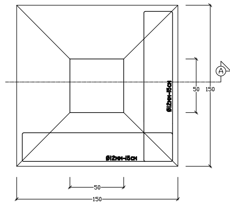
PONDASI FOOT PLAT (FP 150/150) SKALA 1 : 20
