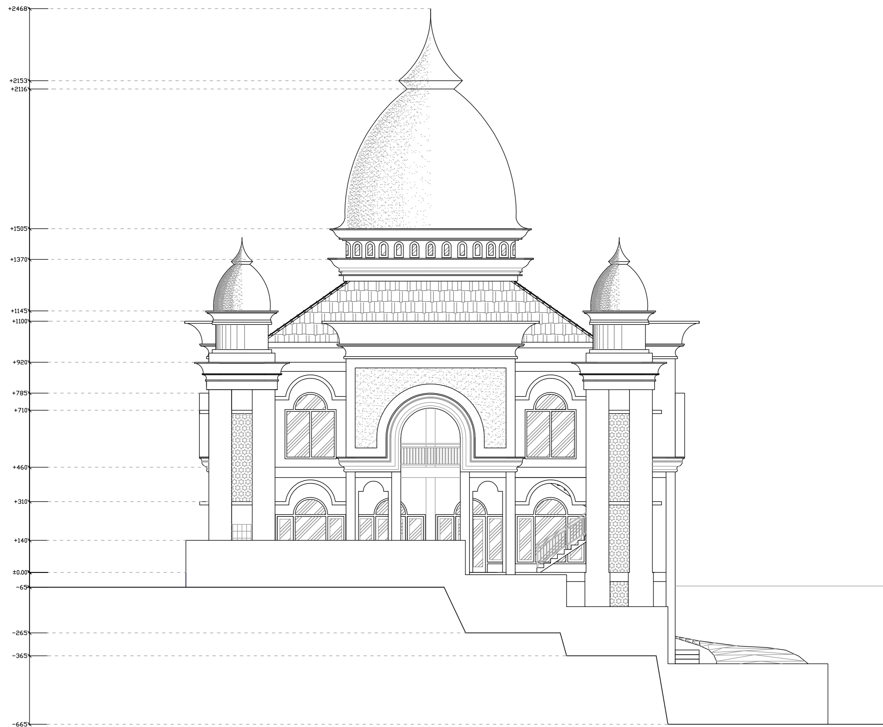
TAMPAK SELATAN SKALA 1 : 100
