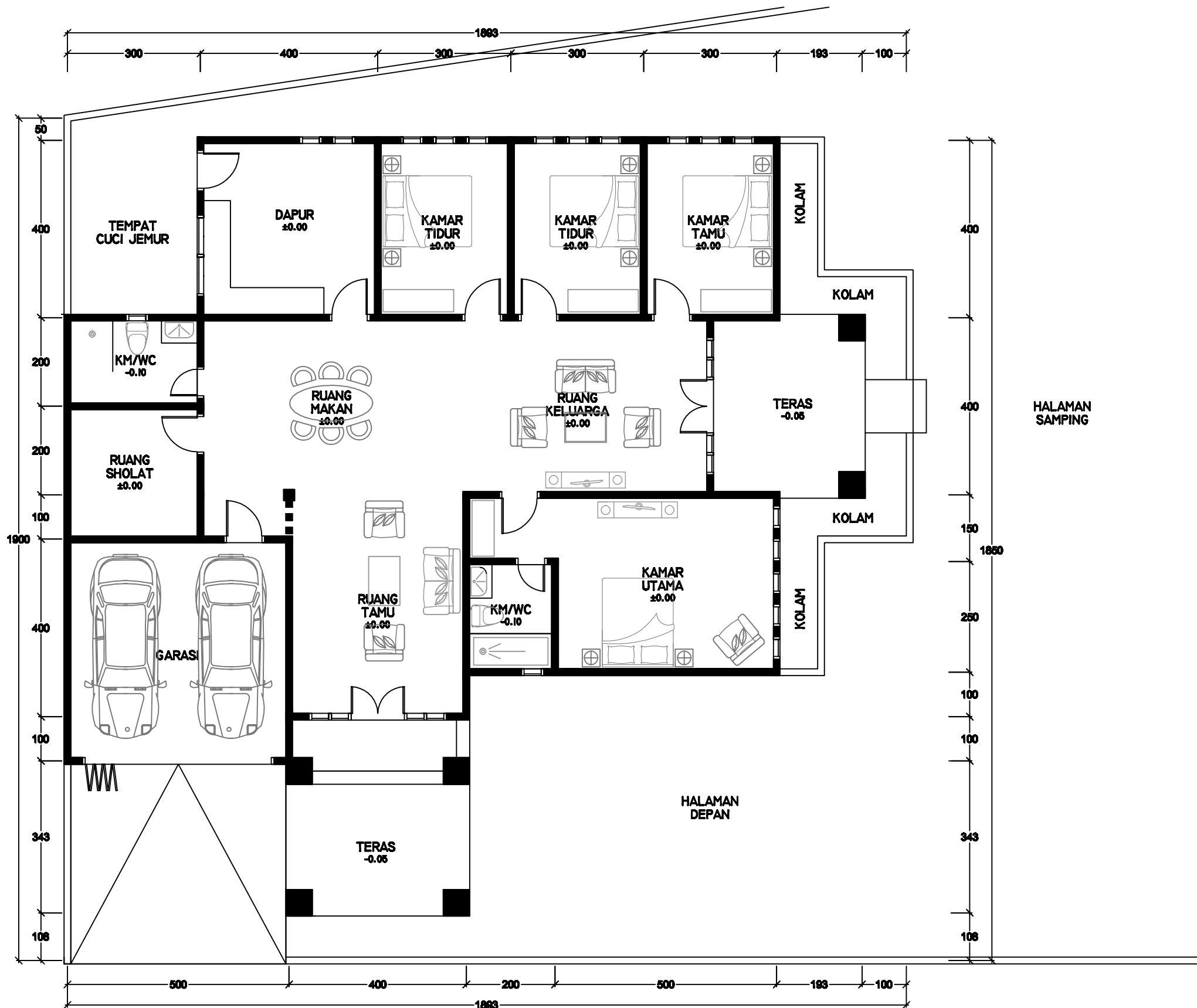
DENAH SKALA 1 : 100
