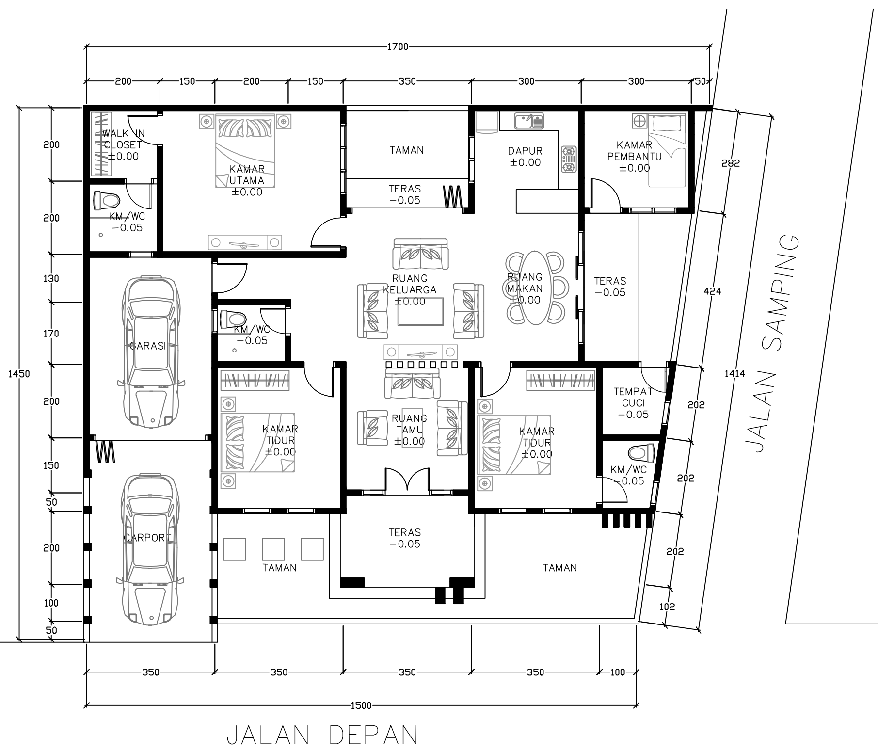
DENAH SKALA 1 : 100
